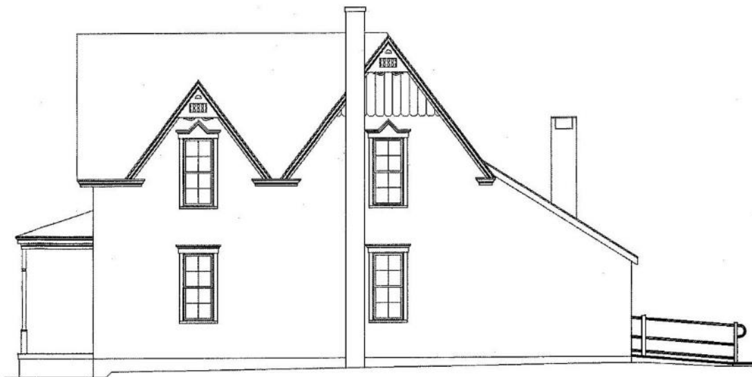
2 RIGHT SDE ELEVATION SCALE: 1/8"=1'-0"
